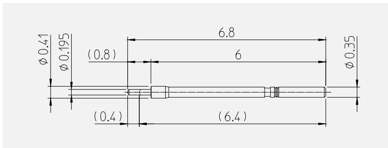
世界最小スプリングコネクターの寸法
