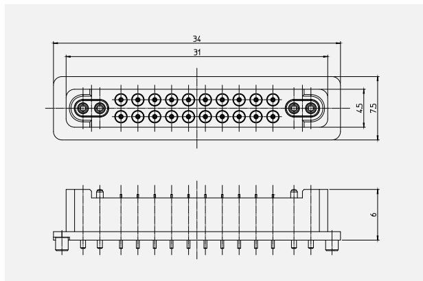
スプリングコネクター
