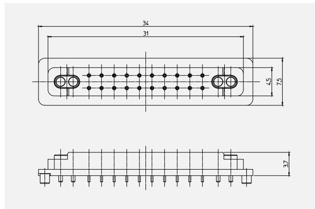
レセプタクルコネクター
